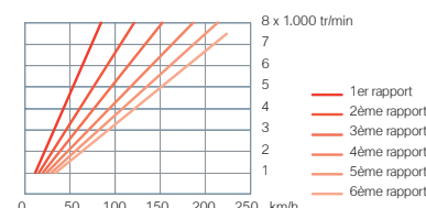
Ce diagramme illustre l'étagement optimal des différents rapports. La boîte de vitesses est dotée d'un sixième rapport court conçu pour une conduite active.
